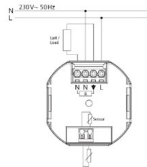
Schaltbildarstellung UTE 4800-R
