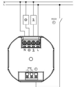
Schaltbilddarstellung UTE 4100-Rw
